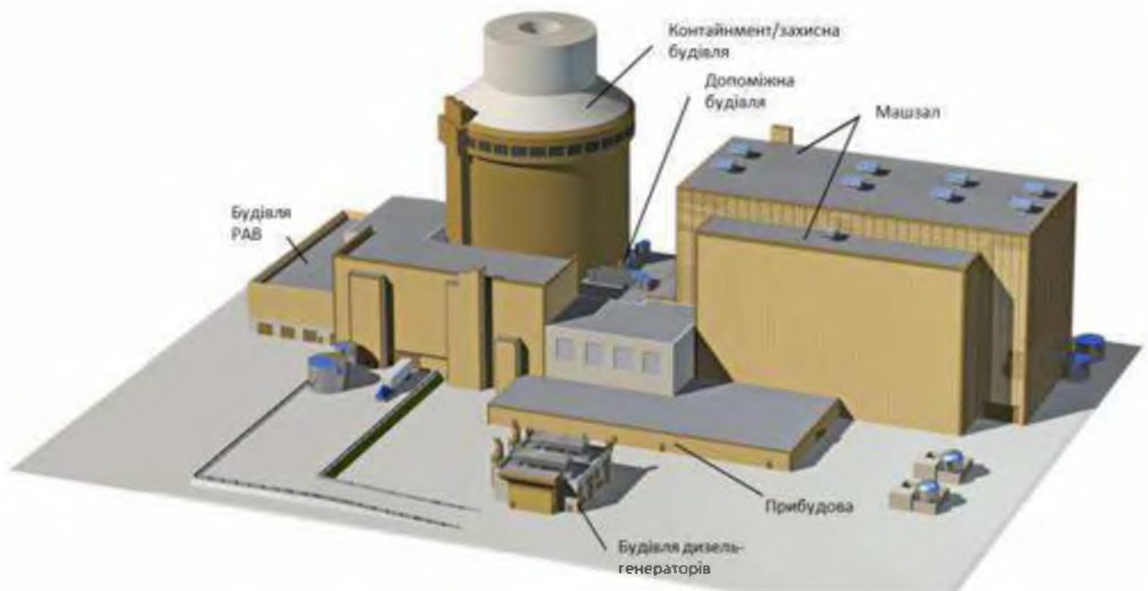
Рисунок 1.2 – Енергоблок AP1000
