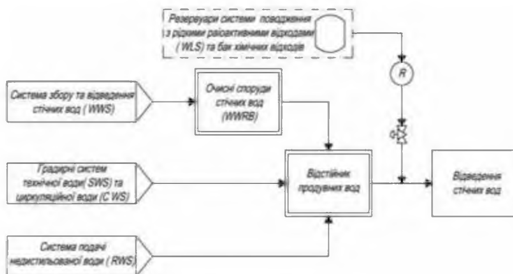
Рисунок 5.3 – Схема відведення стічних вод установки AP1000
