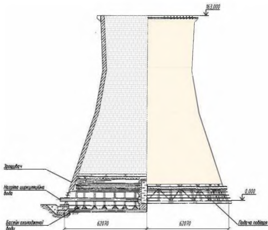
Рисунок 5.1 – Баштова градирня
