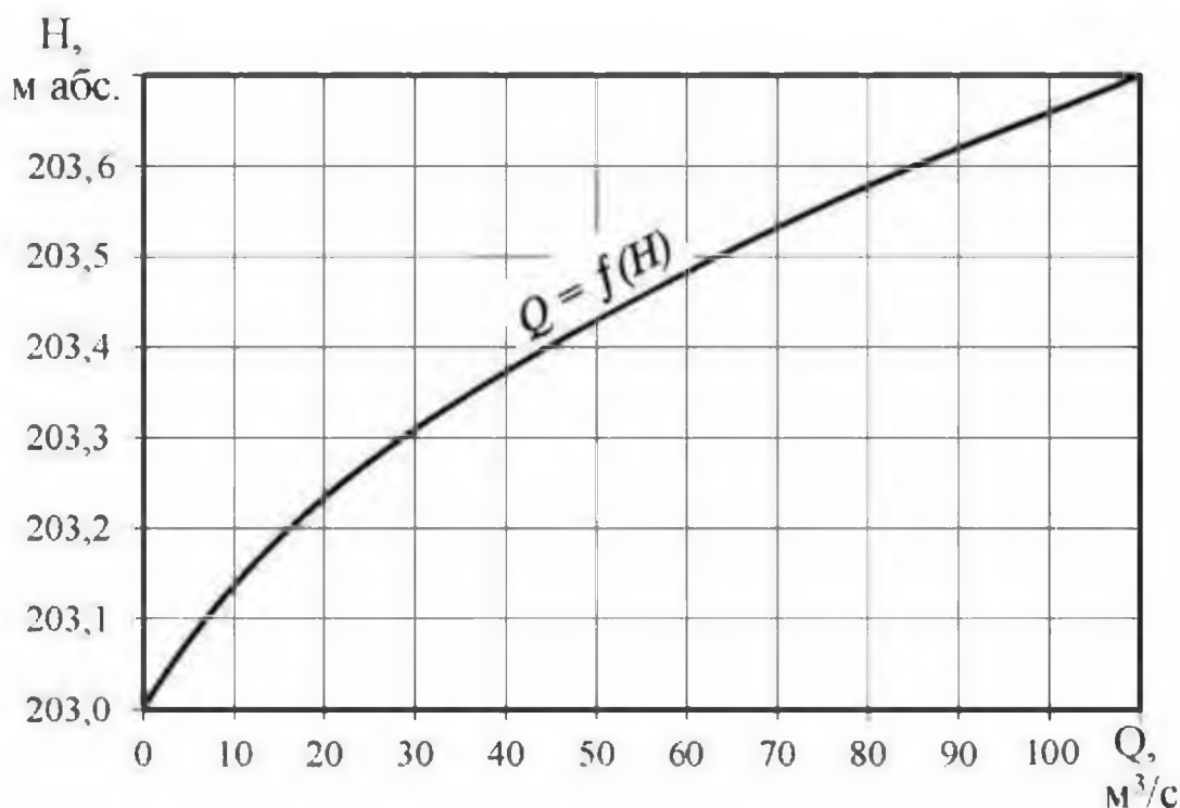
Рисунок 3.6 – Залежність витрат води Q через повеневий водоскид від рівня води H у водоймі охолоджувачі
